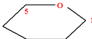
Pyrane réduit
