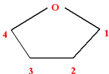
Furane réduit
